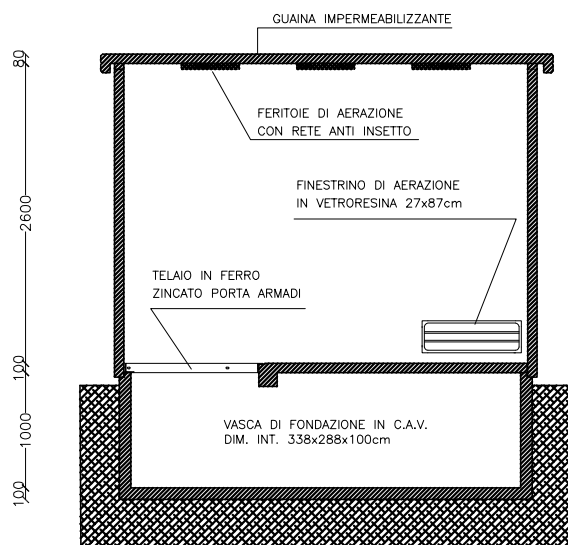
SEZIONE
