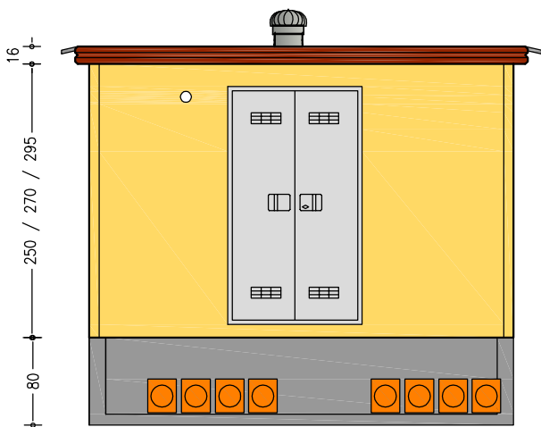
PROSPETTO FRONTALE
