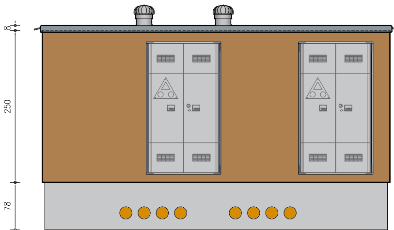
PROSPETTO FRONTALE
