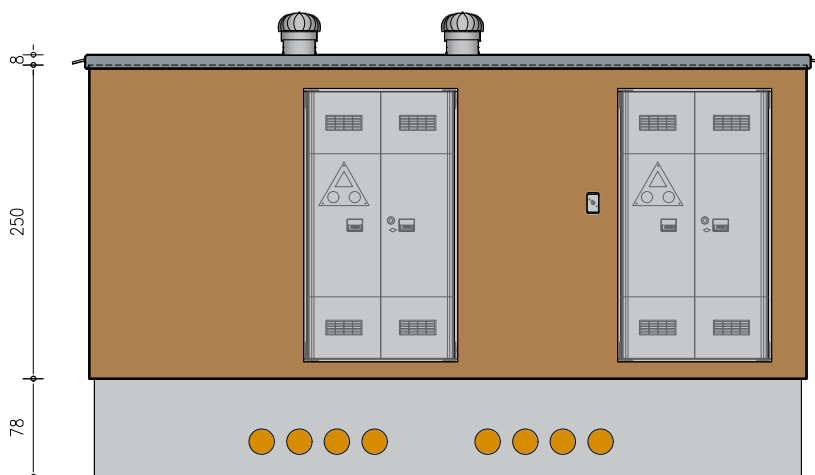
PROSPETTO FRONTALE
