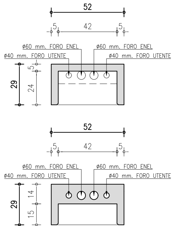
SEZIONI ORIZZONTALI
