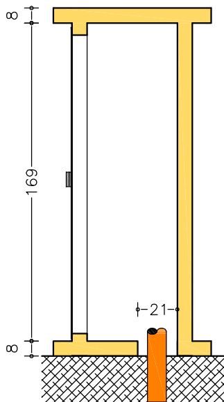
SEZ. B-B
