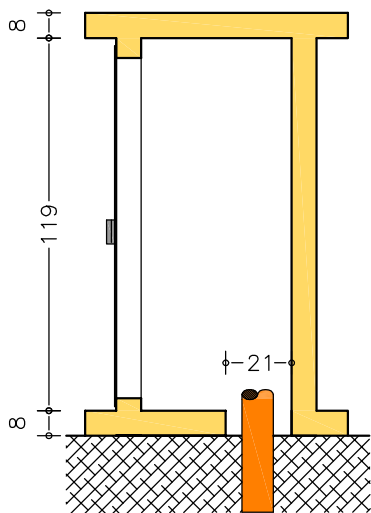
SEZ. B-B
