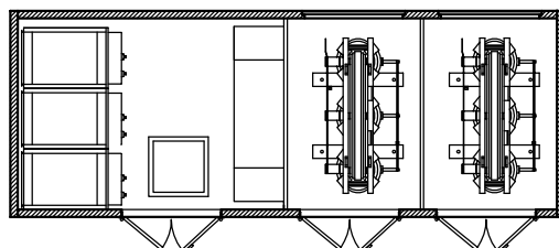
MT-BT / 2TRAF0
