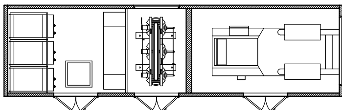
MT-BT / TRAF0 / G.E.
