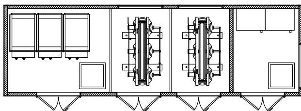
MT / 2TRAF0 / BT
