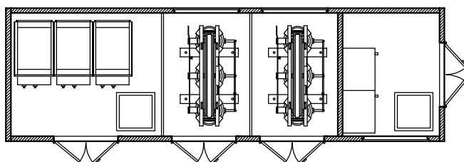
MT / 2TRAF0 / BT 2
