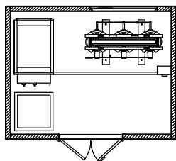
MT / TRAF0
