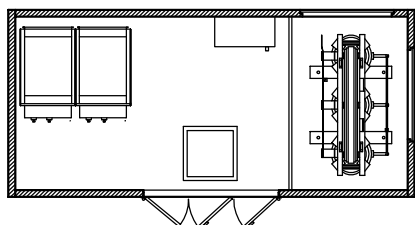
MT-BT / TRAF0
