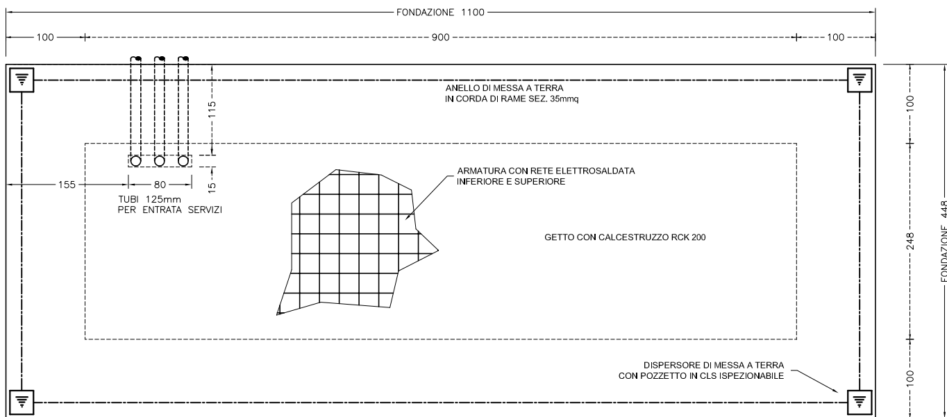
PIANTA FONDAZIONE
