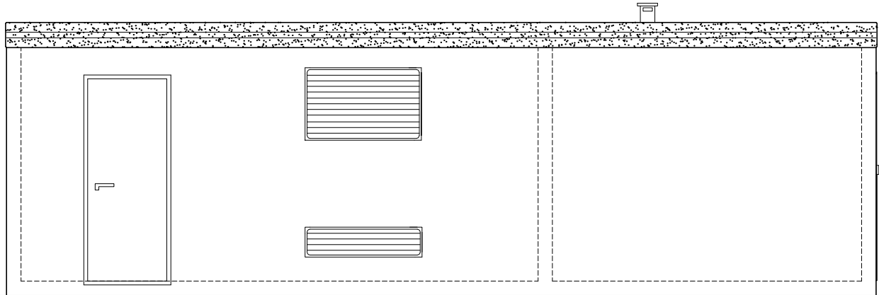
PROSPETTO RETRO
